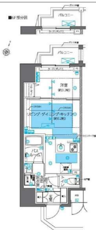
間取り図
