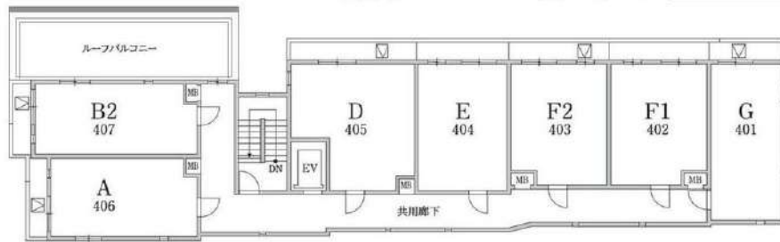
【4階平面図】
